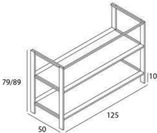
Air 125. Estructura a suelo con dos estantes
